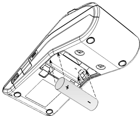
Рисунок 3. Установка аккумулятора
