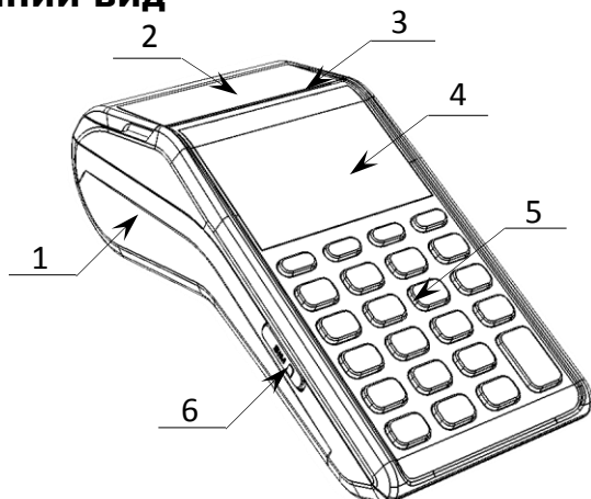
Рисунок 1. Вид спереди/слева
